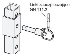
Przykład montażu
